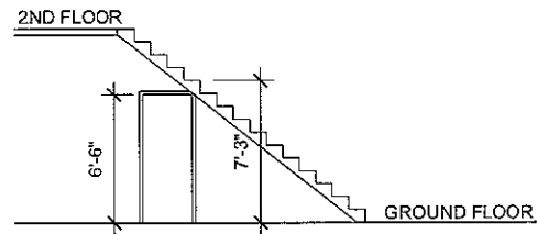
DOOR CLEARANCE
